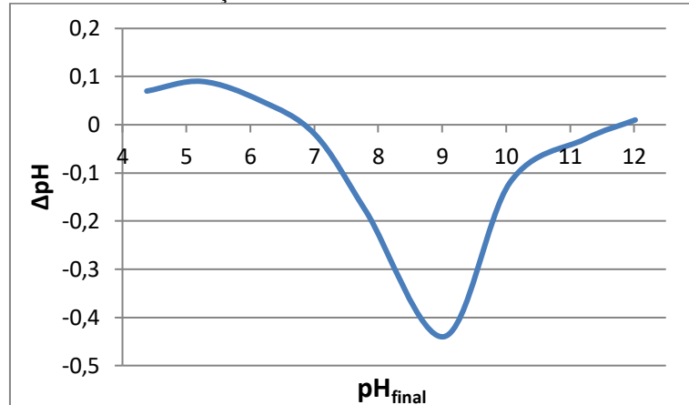
Figura 2 - Ensaio de determinação do PIE da hemimorfita via método de Mular e Roberts.
